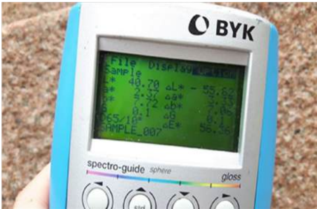
Figura 15. Colorímetro de modelo Spectro Guide Sphere Gloss TR220 da marca BYK..
