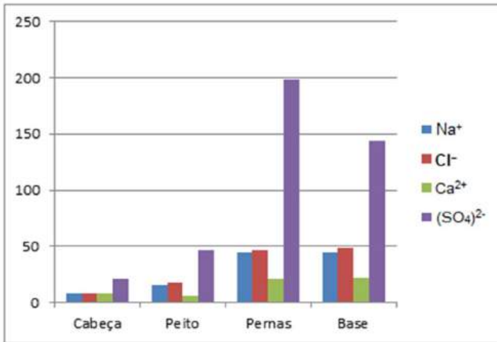
Figura 31. Teores de íons \text{Na}^+ , \text{Ca}^{2+} , \text{Cl}^- e (\text{SO}_4)^{2-} ( \text{mg.L}^{-1} ) em cada ponto avaliado.
