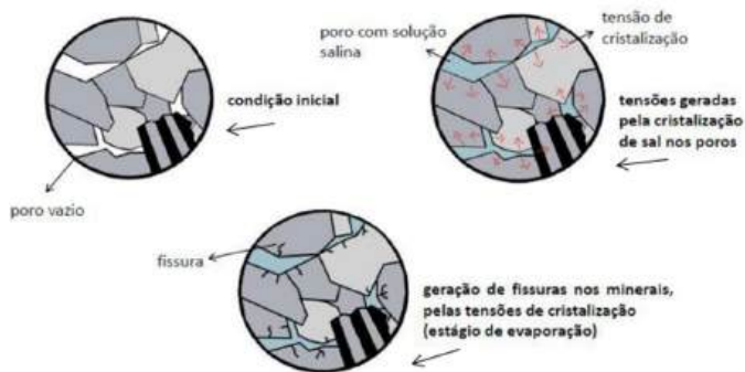
Figura 33. Esquema da percolação e tensões e fissuras geradas pela cristalização de sal em poros de uma rocha. (OLIVEIRA, 2019).
