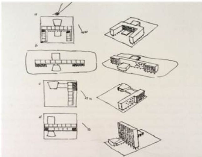
Figura 4. Croquis das propostas para o edifício elaboradas pela equipe de Lucio Costa após o concurso de anteprojetos (representados por Oscar Niemeyer, posteriormente à construção): a) primeiro estudo apresentado pela equipe de Costa; b e c) projetos de Le Corbusier para a Praia de Santa Luzia e Esplanada do Castelo, respectivamente; e d) proposta final elaborada pela equipe de Costa e aprovada por Capanema (MINDLIN, 1956, apud SEGRE, 2013, p. 223).
