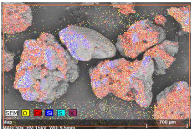
Figura 32. Mapeamento feito pelo MEV/EDS, onde é possível observar acúmulo de cálcio, enxofre e oxigênio dando origem à cristais de gipsita ( \text{Ca}(\text{SO}_4) \cdot 2\text{H}_2\text{O} ).
