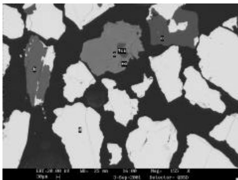
Figura 3 - Imagem do minério de barita, onde (a) - feldspato rico em bário, (b) e (e) - mica (provável biotita), (c) - quartzo e (d) - barita. MEV/BSD.
