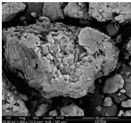
Figura 5. Imagem da amostra bentonita clara (MEV). Elétrons retroespalhados.
